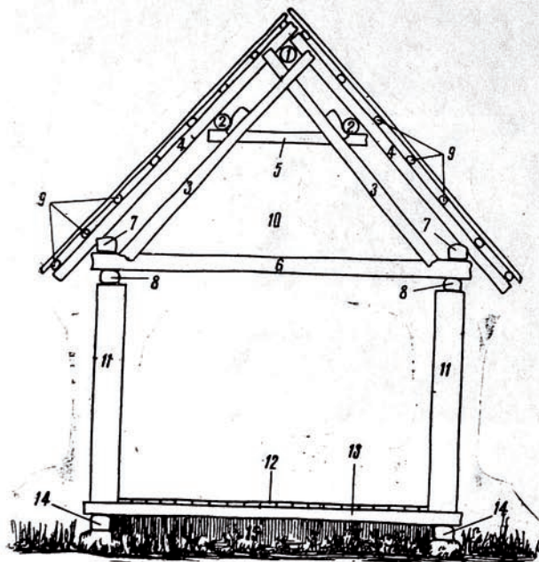
41-чи шәкил. Гутгашен районунун Һәзрә кәнди, евин кәсији; 1—баш тир; 2—гуршаг; 3—сипо; 4—гож саллама; 5—замын (тоуг-јатан); 6—сипо пәрдис; 7—гара тир; 8—сүтун пәрдис; 9—пүштөван; 10—дам; 11—сүтун пәрдис; 12—дөшәмә; 13—јер пәрдис; 14—дивар; 15—каналты (дамчыдөјөн).
