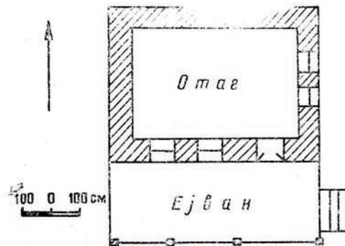
38-чи шәкил. Варташен рајонунун Хачмаз кәнд сакини М. Газыјевини јени тикдирдији јашајыш еви (1966-чы ил).
