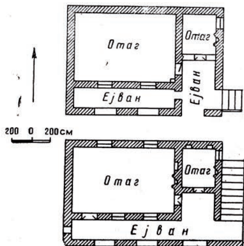
21-чи шәкил. Загатала районунун Биринчи Тала кәнд сакини Ч. Һ. Ага-Јевни икимәртәбәли јашајыш еви
