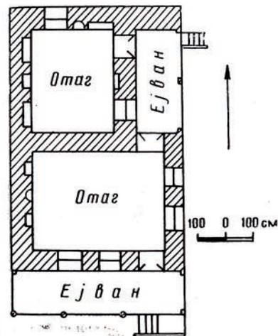
27-чи шәкил. Варташен районунун Хачмаз кәнд сакини Н. М. Әфәнди- нин јашајыш еви (1966-чы ил).
