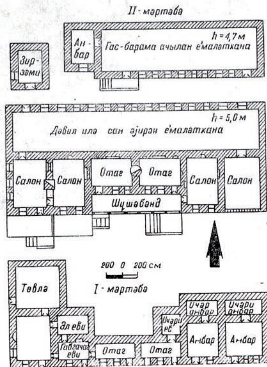
36-чы шәкил. Шәки шәһәр сакини М. Начырасул оғлунун јашајыш еви вә ипәк е'малатханасы планы (1966-чы ил).
