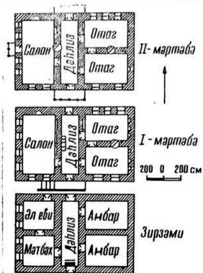
33-чү шәкил. Шәки шәһәр сәкинн ш. Б. Шихалиевни јашајыш еви (1966-чы ил).
