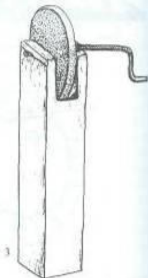
XXI tablo. Dəmirçi alət və ləvazimatı: 1 – Zindan kütəyi, düzbocaq, tayqulaq və qosaqulaq zindanlar, eşək, möhtir; 2 – Qosaqitlik işlək halda; 3 – Xarı dəsi.
