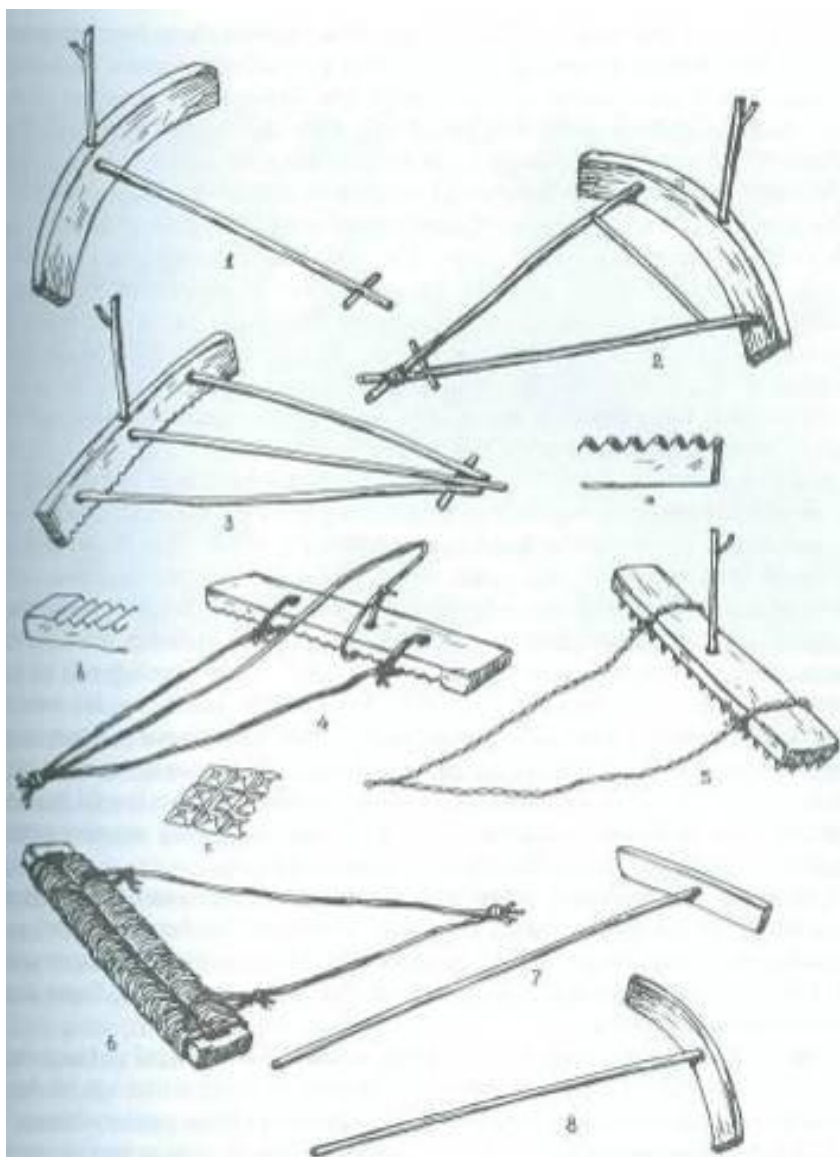
Lankaran-Astara bölgəsində çətikçilikdə işlənilən çətik malaları: 1, 2 – peskovit mala; 3 – giranda mala; 4 – çaqa mala; 5 – dişli mala; 6 – bamar-toxuma mala; 7, 8 – dastirandli (ol malası); a, b, c – malaların işlək hissələri
