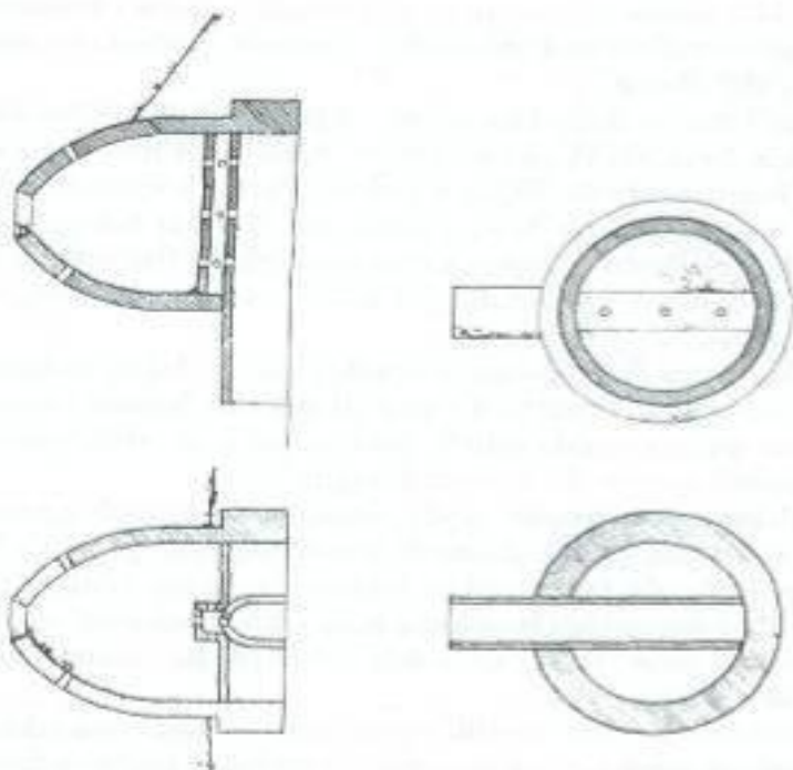
X tablo. Dulus sobasi. Quba rayonunun Yenikend kəndi.
