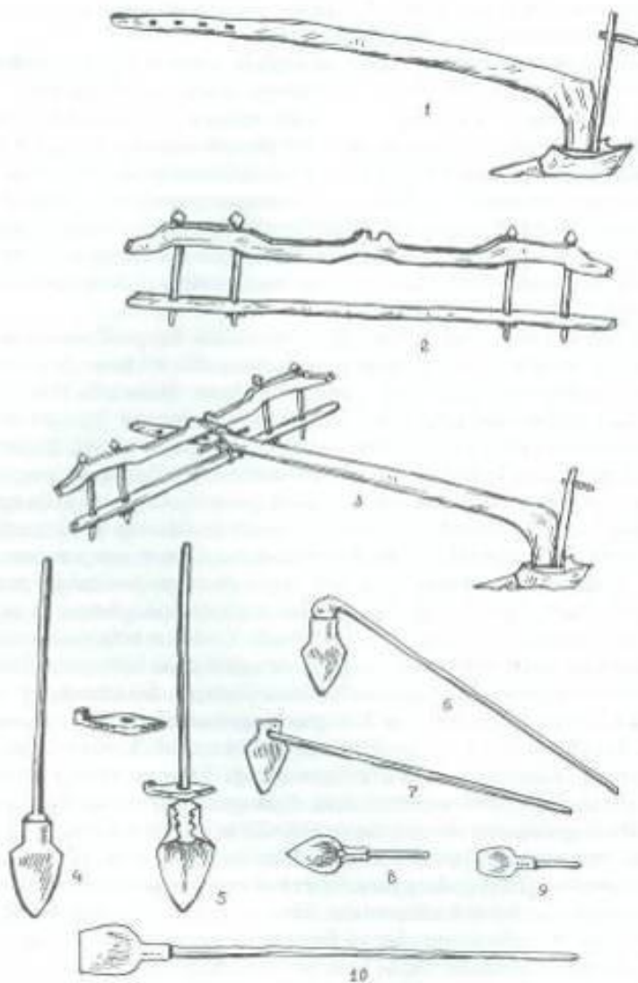
Lankaran-Astara bölgəsində çalığıçılıqda işlədilan şum alətləri: 1 - çalığı oxu; 2 - giv-boyunducu; 3 - xısalat; 4, 5 - bel; 6, 7 - ayrı bel; 8, 9 - belça; 10 - tuncar bel
